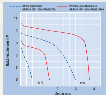
Spannungsverläufe geschlossener Batterien NBB 248 12V 125 Ah und verschlossener Bleibatterien „dryfit“ NBB 248 12V 100 Ah bei Belastung mit 500 A bei -30 °C und 0 °C nach 16 h Konstantspannungsladung mit 14,4 V.
